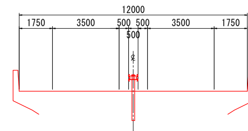
橋梁部 (長大橋)
