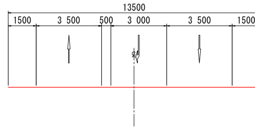
交差点部 (起点部)
