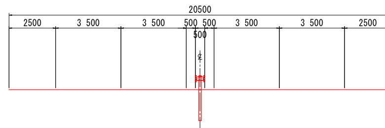
付加車線部 (切土部)
