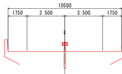
橋梁部 (起点部)
