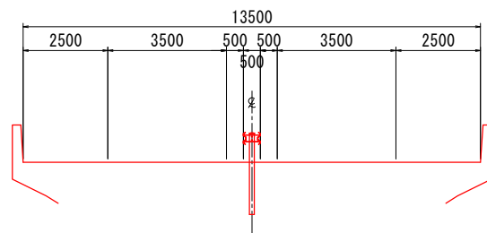
橋梁部 (中小橋)
