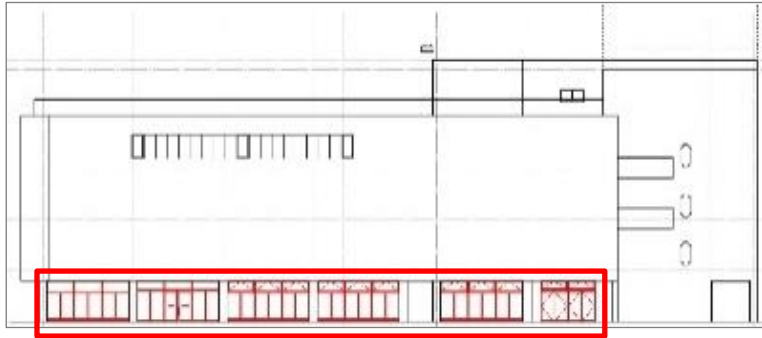
南側立面図
