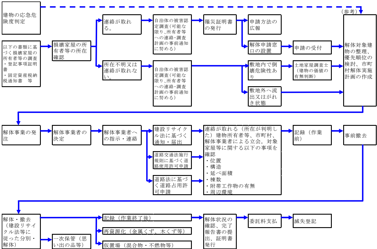
図6-6 撤去等フロー（参考：対策指針）
