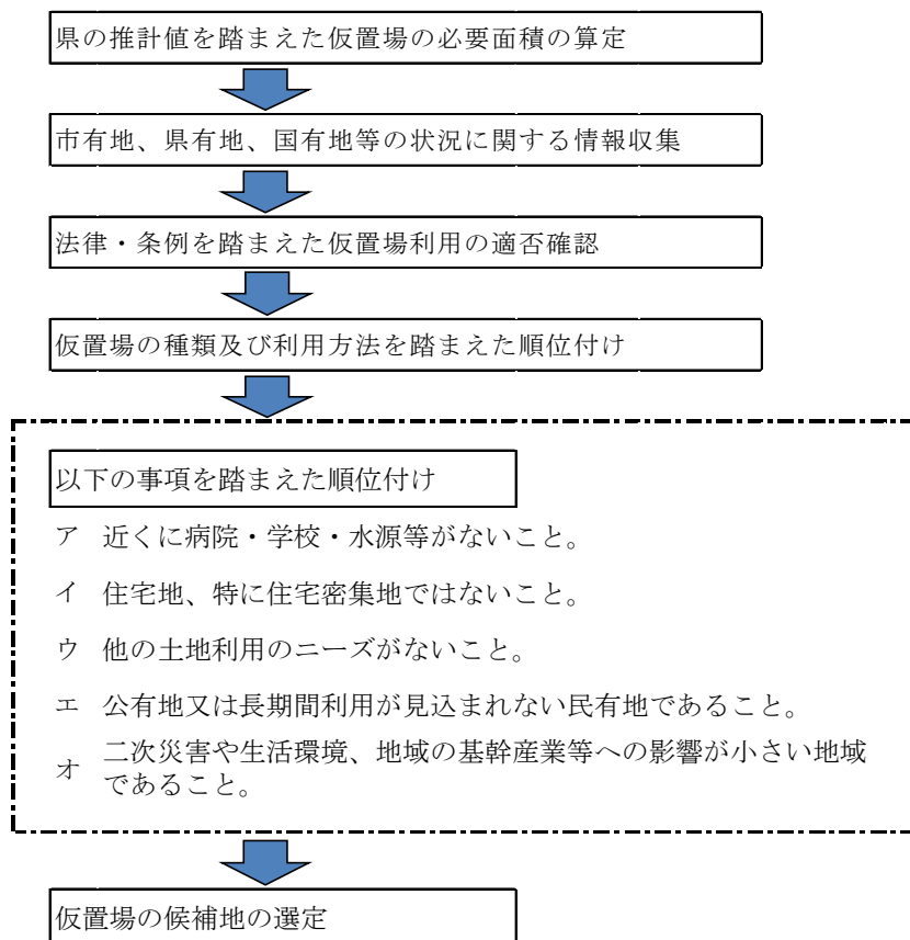
図6-1 仮置場の選定フロー（要件等）（参考：対策指針）
