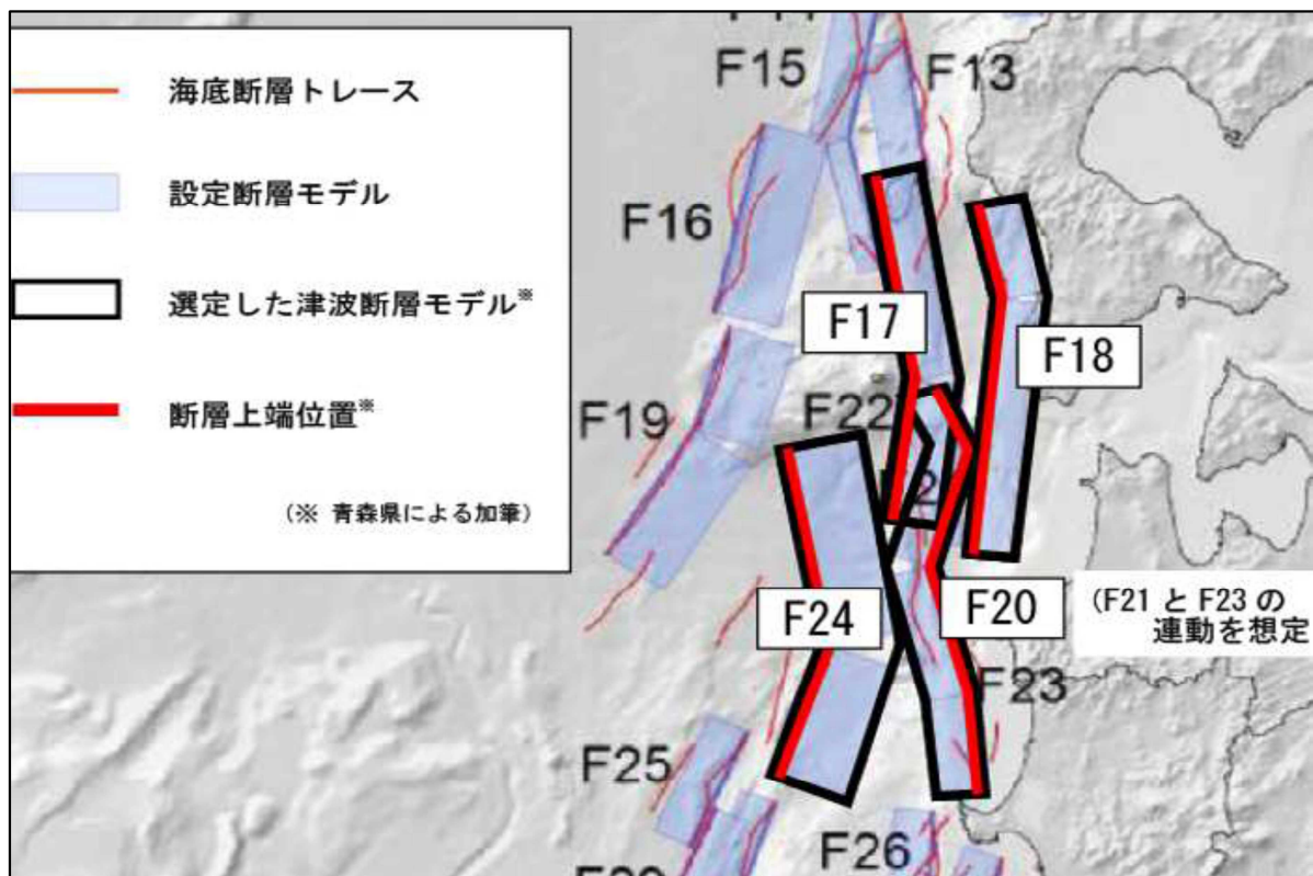
図4-2 平成27年度青森県地震・津波被害想定調査における震源モデル (参考：青森県地域防災計画 地震・津波災害対策編)
